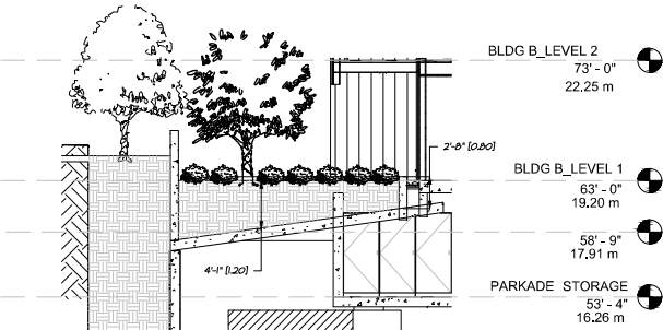
01 SECTION 6 L20 SCALE: 3/16"=1'-0"
