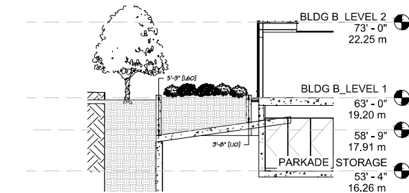
02 SECTION 7 L20 SCALE: 3/16"=1'-0"
