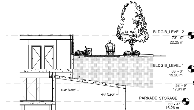
05 SECTION 5 L19 SCALE: 3/16"=1'-0"
