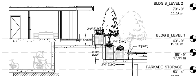
02 SECTION 2 L19 SCALE: 3/16"=1'-0"
