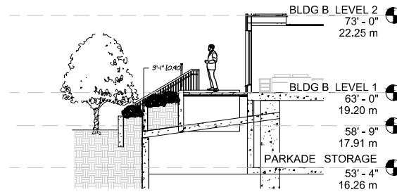
03 SECTION 8 L20 SCALE: 3/16"=1'-0"
