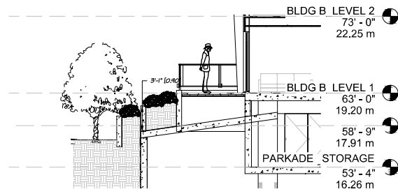
04 SECTION 9 L20 SCALE: 3/16"=1'-0"
